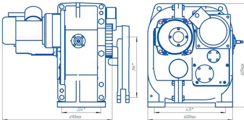
Габаритные размеры механизмов МЭО- 4000-ИВТ4Gb
